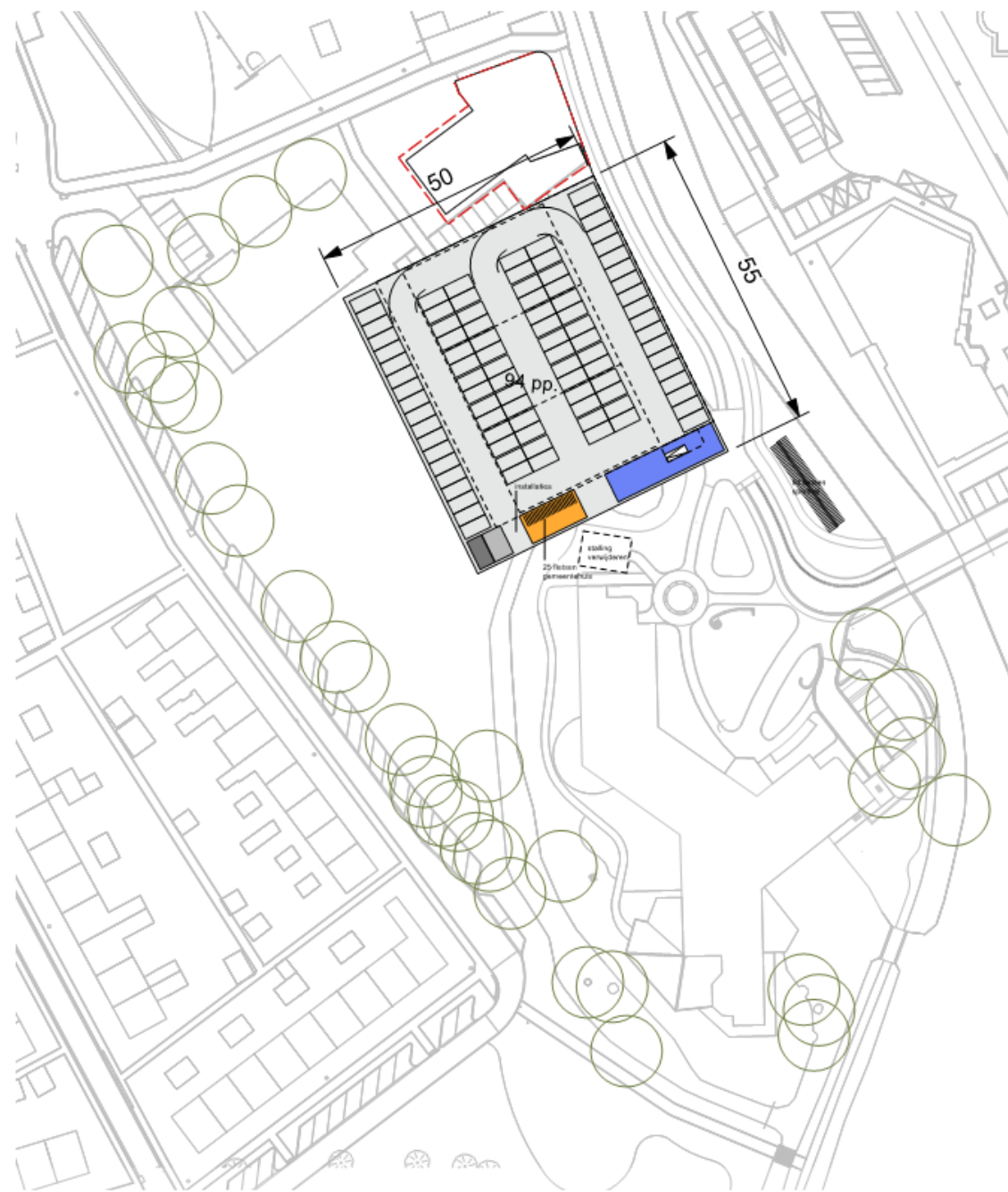
Begane Grond
